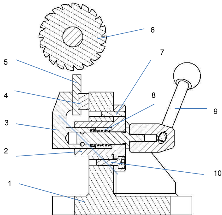
1 Grundkörper; 2 Buchse; 3 Spannhaken; 4 Auflagestück; 5 Werkstück; 6 Scheibenfräser; 7 Zylinderstift; 8 Druckfeder; 9 Spannhebel M10; 10 Zylinderschraube
