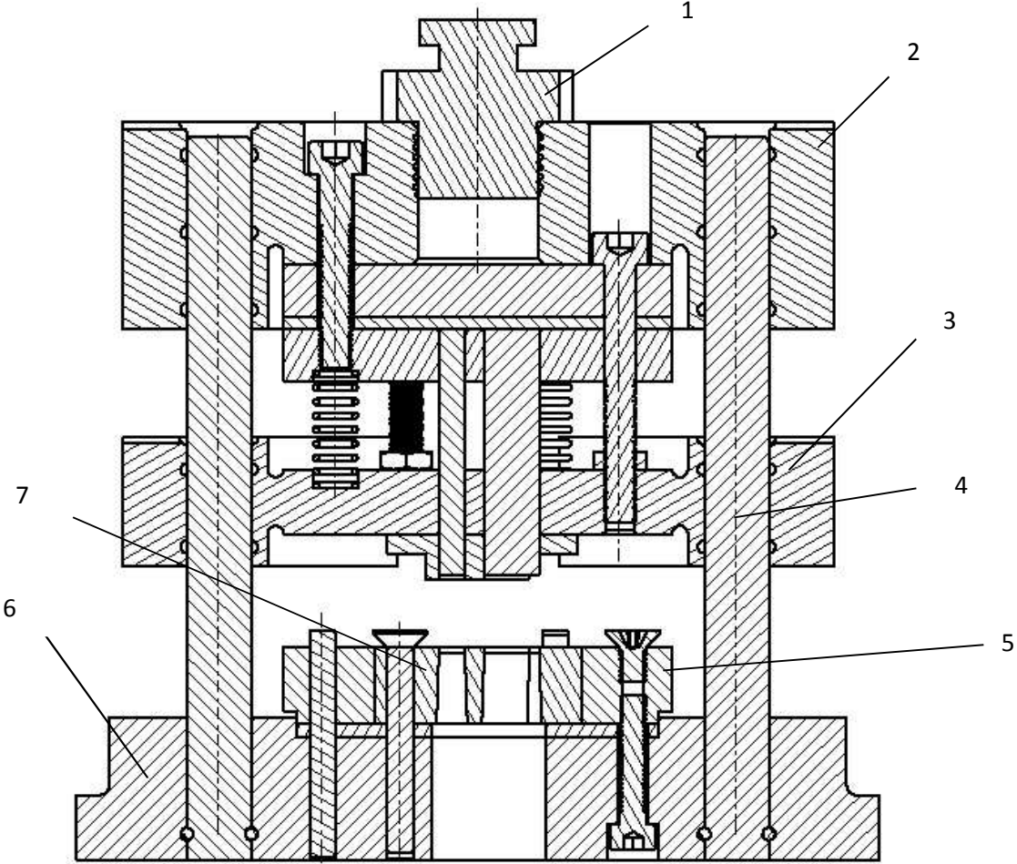
1 Einspannzapfen; 2 Gestell oben; 3 Auswerferplatte; 4 Führungssäule; 5 Aufnahmeplatte unten; 6 Grundplatte; 7 Schneideinsatz
