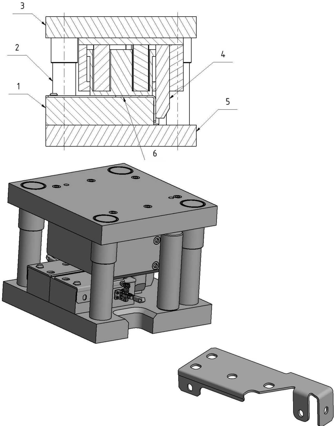
Bild 2-30 Biegewerkzeug für Haltewinkel 1 Zentrierplatte fürs Werkstück; 2 Führungssäule; 3 Kopfplatte; 4 Biegestempel; 5 Grundplatte; 6 Werkstück Haltewinkel
