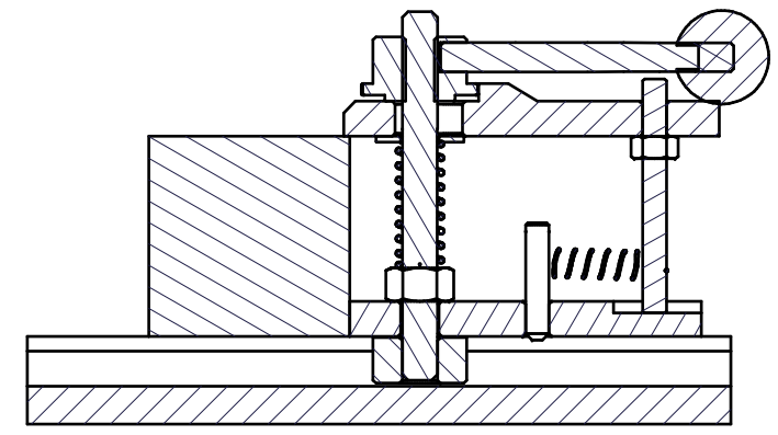
A-A (1:1)
