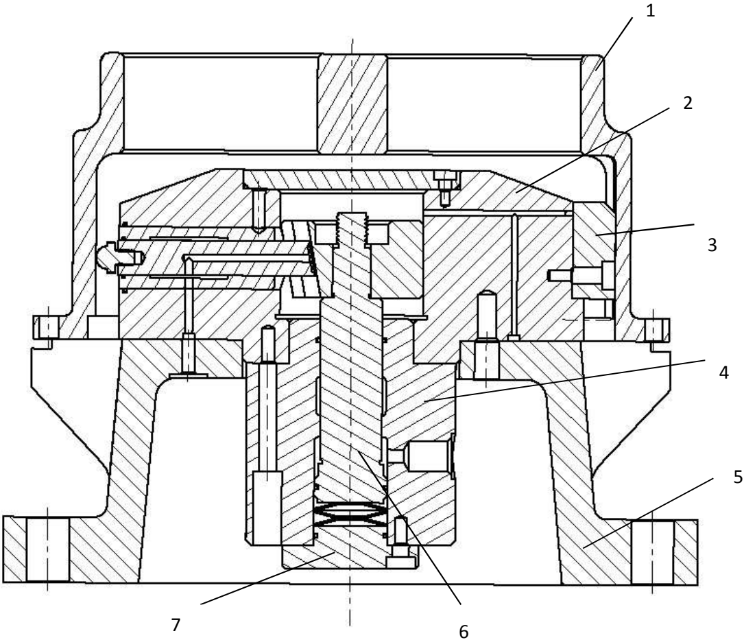
1 Werkstück; 2 Vorrichtungskörper 3 Zentrierstück; 4 Kolbengehäuse ; 5 Vorrichtungskörper unten ; 6 Kloben; 7 Deckel für Kolbengehäuse;
